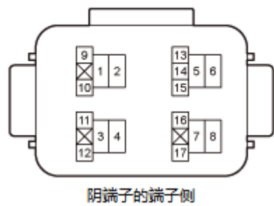
辅助发动机盖下继电器盒 B 的 17 针插座
